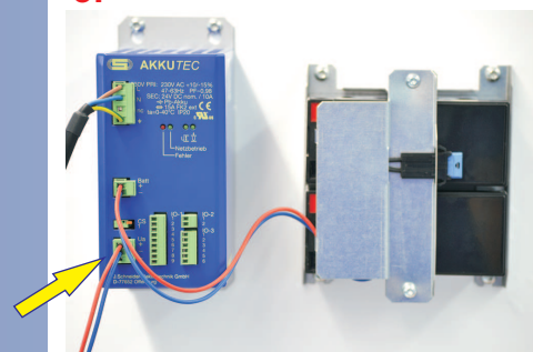
Anschluss der Last an den gepufferten 24 V DC Ausgang des AKKUTECH
