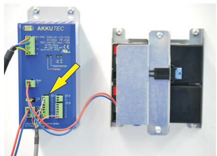
Anschluss des RS232 Schnittstellenkabels (Art. Nr. PSDP0324G0100X)
