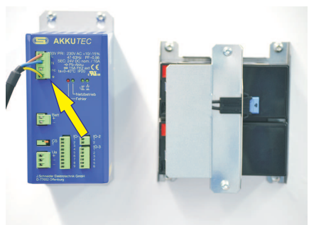
Anschluss des AKKUTECH an das Versorgungsnetz (230 V AC)
